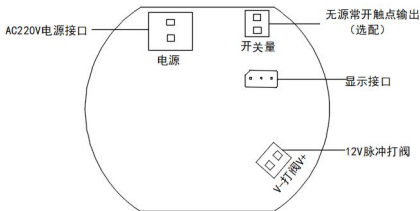
图 4-2 接线示意图
