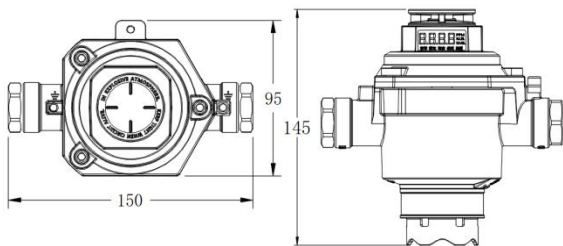
图 2-1 外形尺寸示意图（单位：mm）
