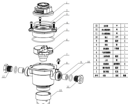
图 2-2 组成结构示意图
